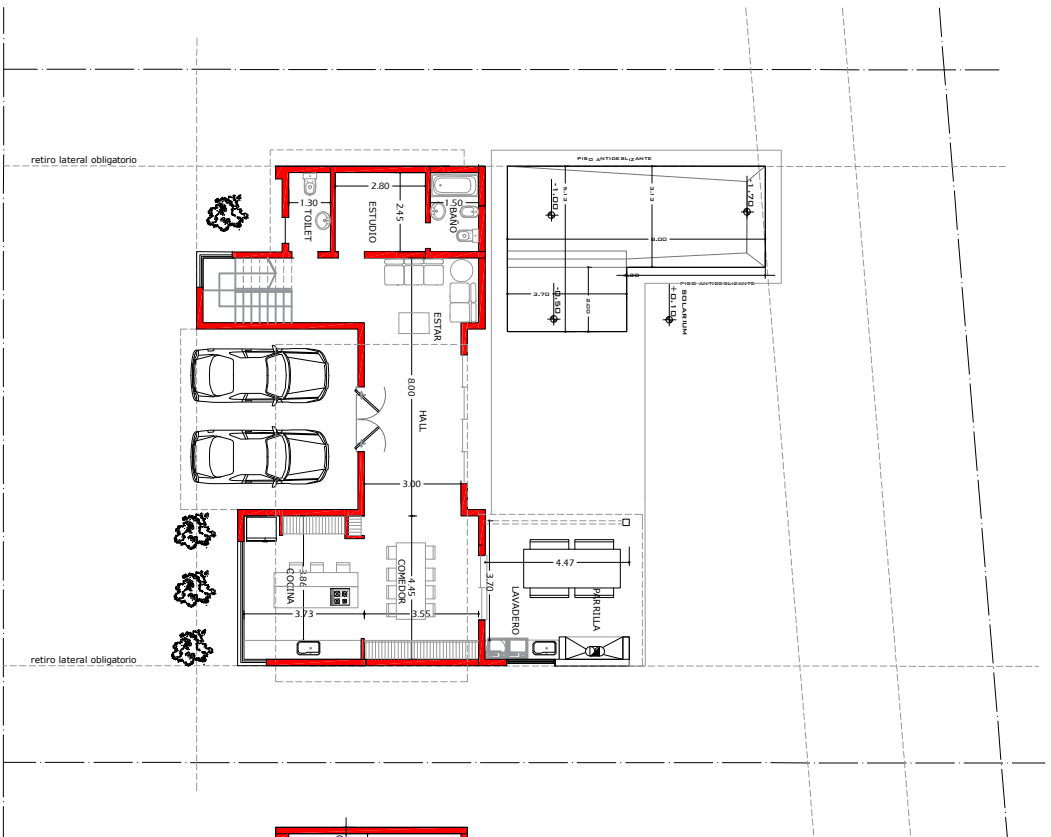
PLANTA BAJA Esc.:1:100
