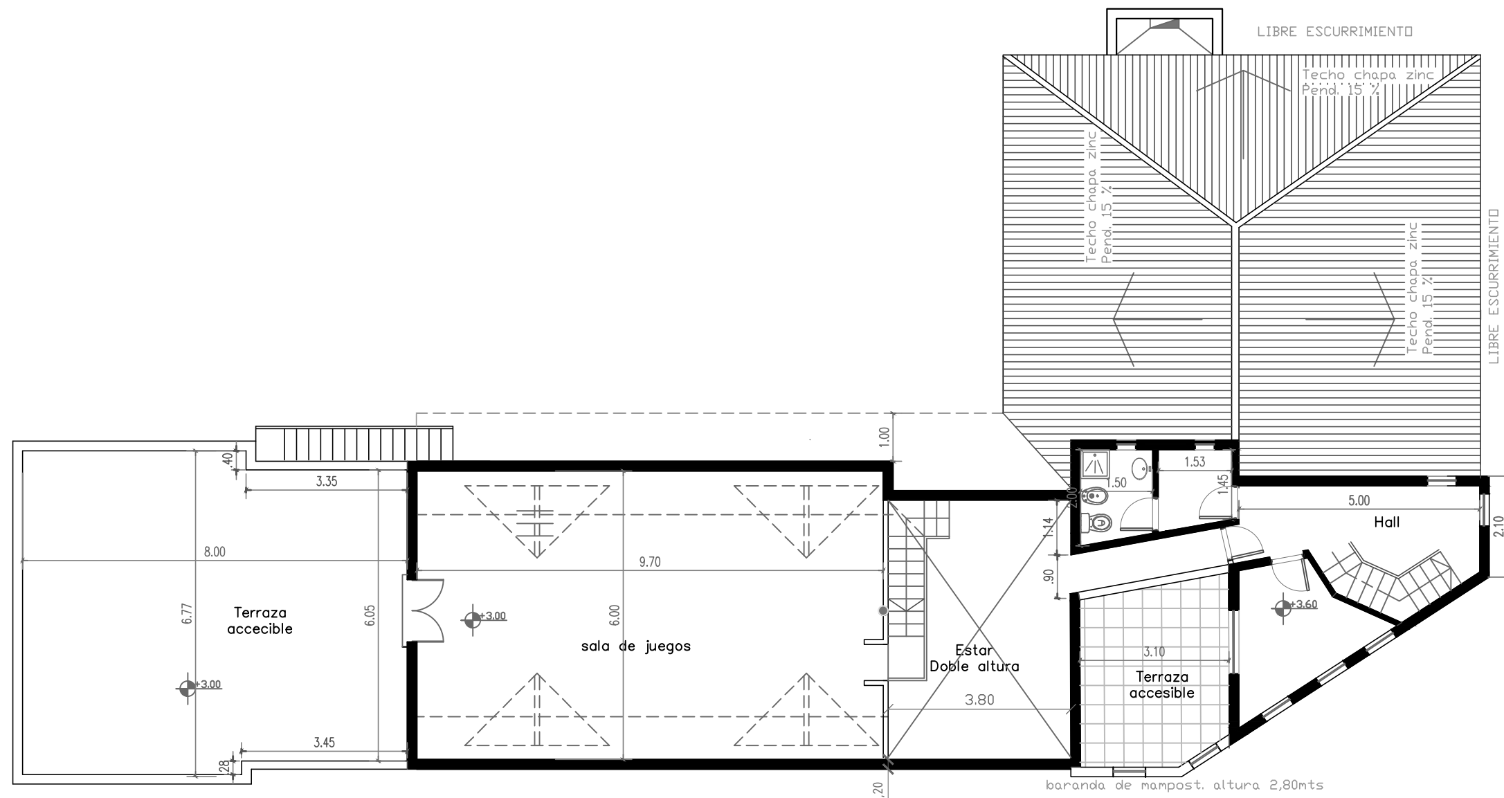
PLANTA ALTA
