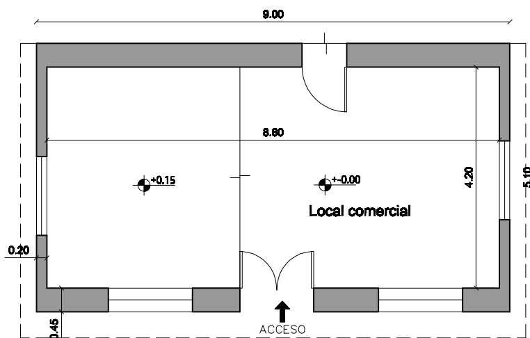
PLANTA LOCAL COMERCIAL E.S.C: 1:100
