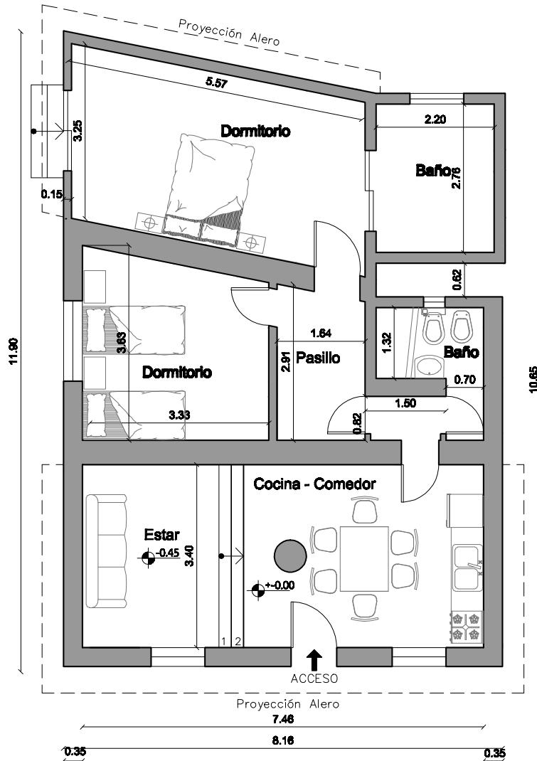
PLANTA VIVIENDA UNIFAMILIAR E.S.C: 1:100
