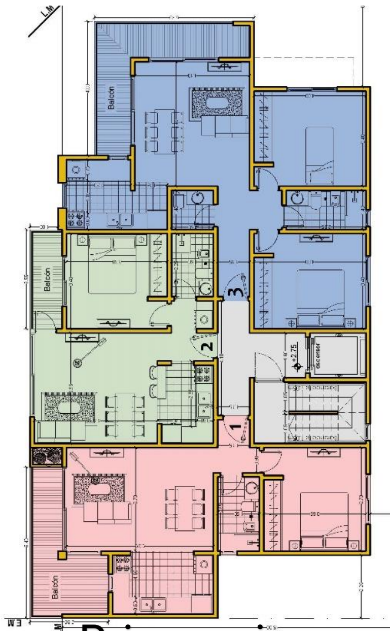
Primer piso
